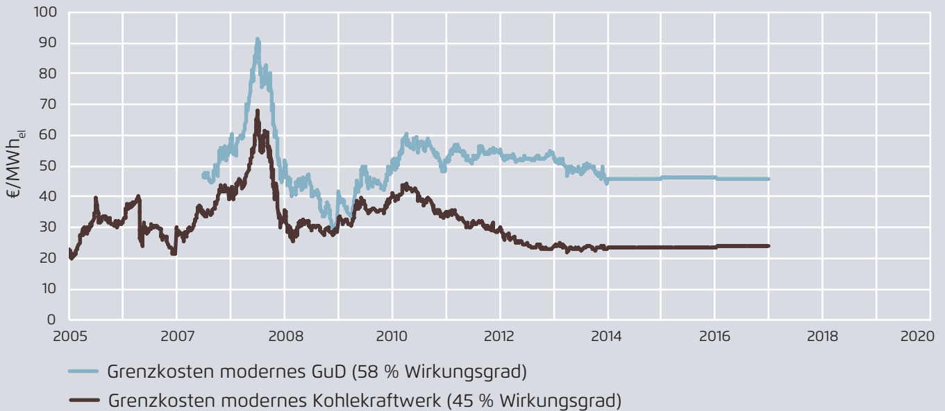
Teures Gas und billige Kohle – Entwicklung der Grenzkosten von Referenzkraftwerken auf Grundlage von Terminmarktprodukten für das jeweils folgende Lieferjahr
