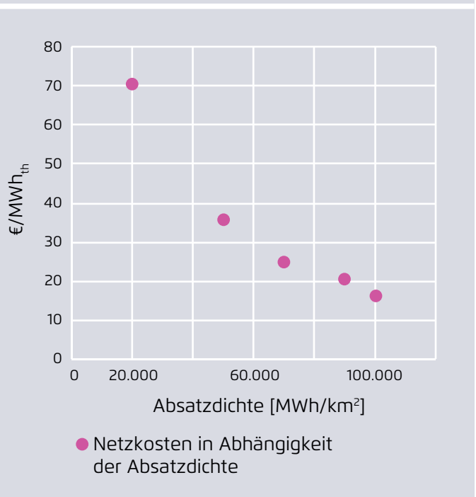
Hohe Netzkosten bei geringer Absatzdichte im Versorgungsgebiet Abbildung 24
