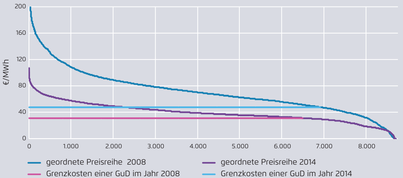
Gesunkene Nutzungsstunden für Erdgas-KWK-Anlagen
