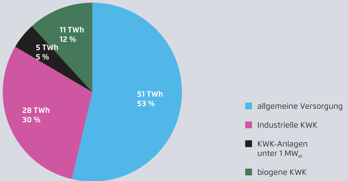
Allgemeine Versorgung und Industrie dominieren die KWK-Stromerzeugung: Anteile an der KWK-Strommenge im Jahr 2012
