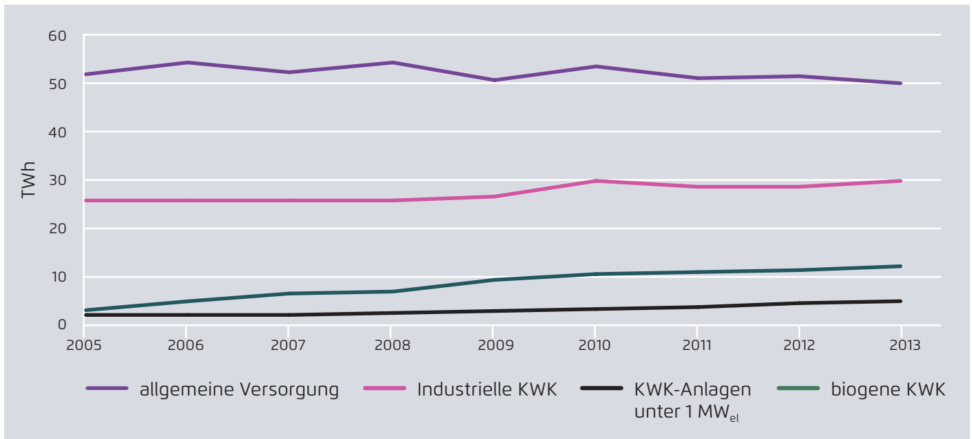
Stagnation der Fernwärme-KWK, Zuwächse in den übrigen Bereichen
