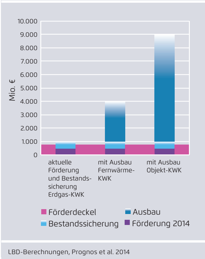
KWK-Fördervolumina bei Bestandssicherung sowie bei zusätzlicher 25-Prozent-Zielerreichung mittels Fernwärme- beziehungsweise Objekt-KWK Abbildung 15
