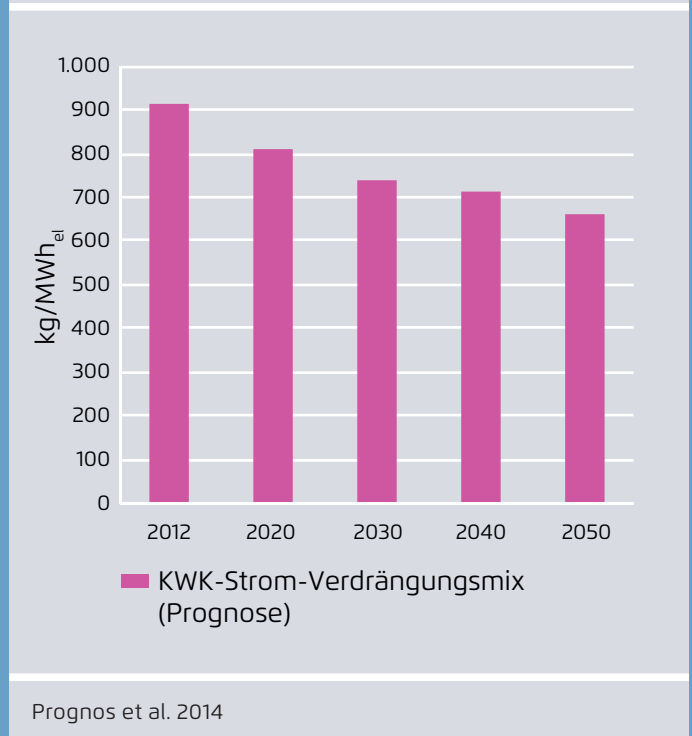
Entwicklung der spezifischen Emissionen im KWK-Verdrängungsmix Abbildung 17
