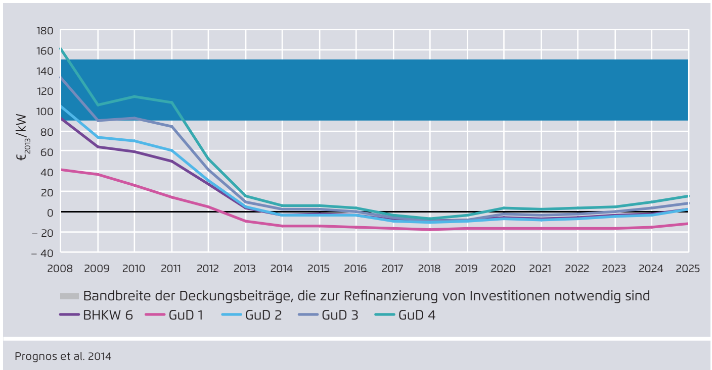
Trotz KWK-Zuschlag weisen viele gasgefeuerte Fernwärme-KWK-Anlagen einen negativen Deckungsbeitrag 2 auf und sind stilllegungsgefährdet
