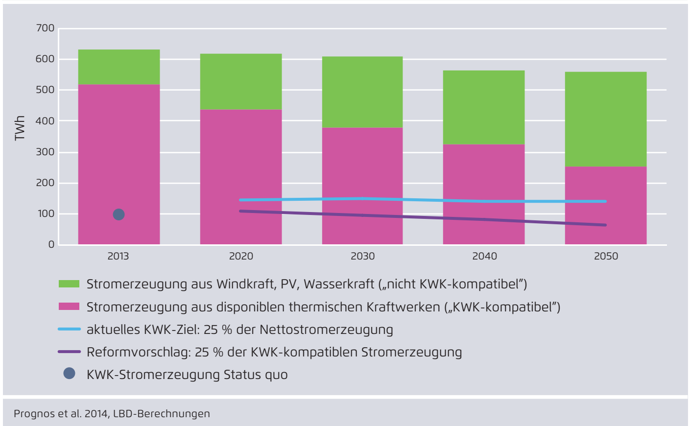
Neudefinition des KWK-Ziels gemäß Prognos et al. 2014: Statt 25 Prozent der gesamten nun 25 Prozent der disponiblen („KWK-kompatiblen“) Stromerzeugung
