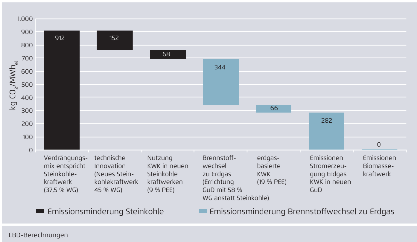
Verschiedene Beiträge zur Emissionsvermeidung thermischer Kraftwerke: Verbesserungen des Wirkungsgrades (WG), Brennstoffwechsel und Primärenergieeinsparungen (PEE) durch KWK
