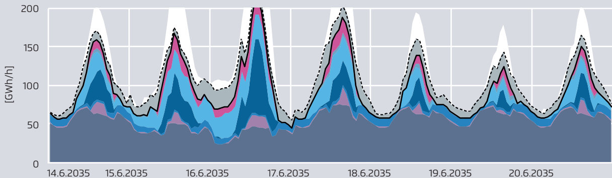
Stündliche Stromnachfrage mit flexiblen Verbrauchern (oben) und bei geringer Flexibilisierung (unten)
