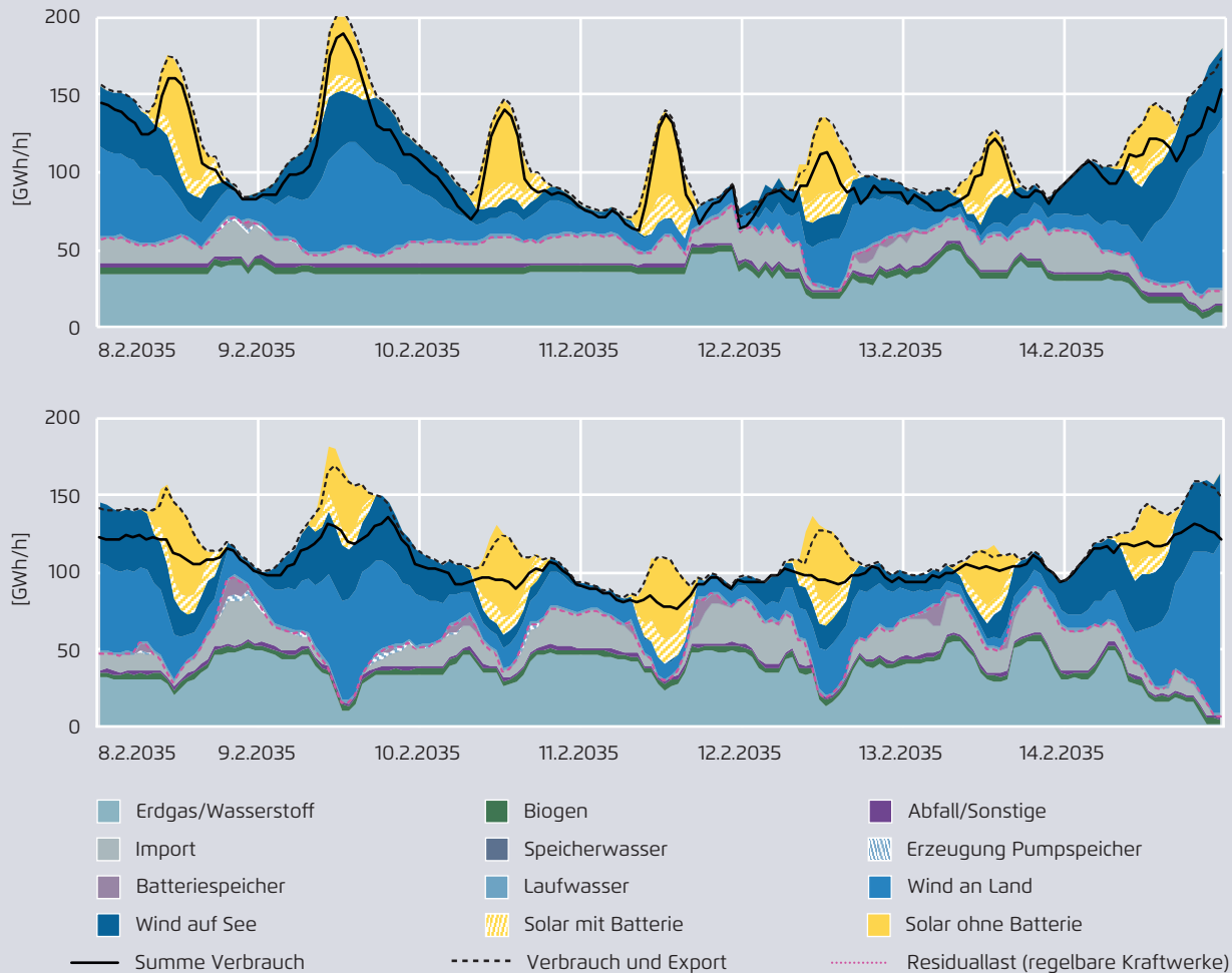
Stündliche Stromerzeugung mit flexiblen Verbrauchern (oben) und bei geringer Flexibilisierung (unten)
