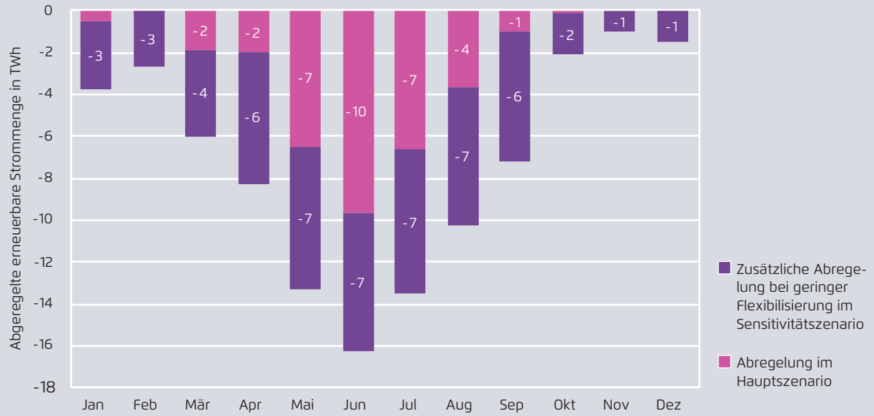
Monatliche Abregelung im Hauptszenario und bei geringer Flexibilisierung
