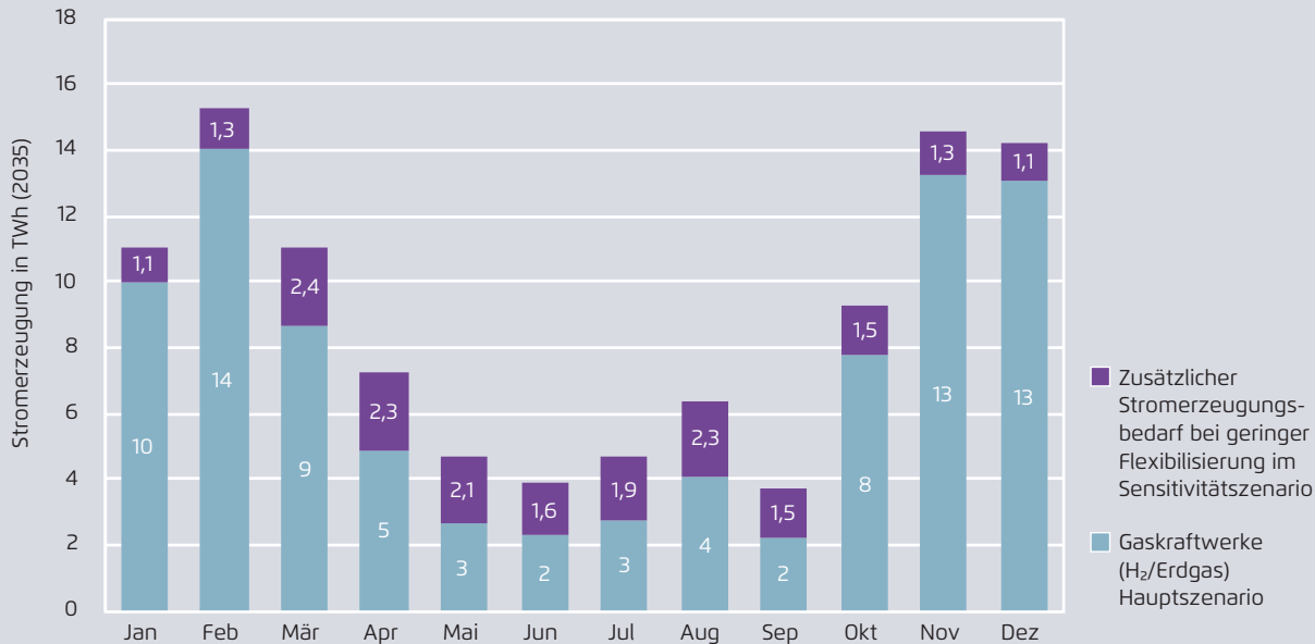
Monatliche Stromerzeugung im Hauptszenario und bei geringer Flexibilisierung
