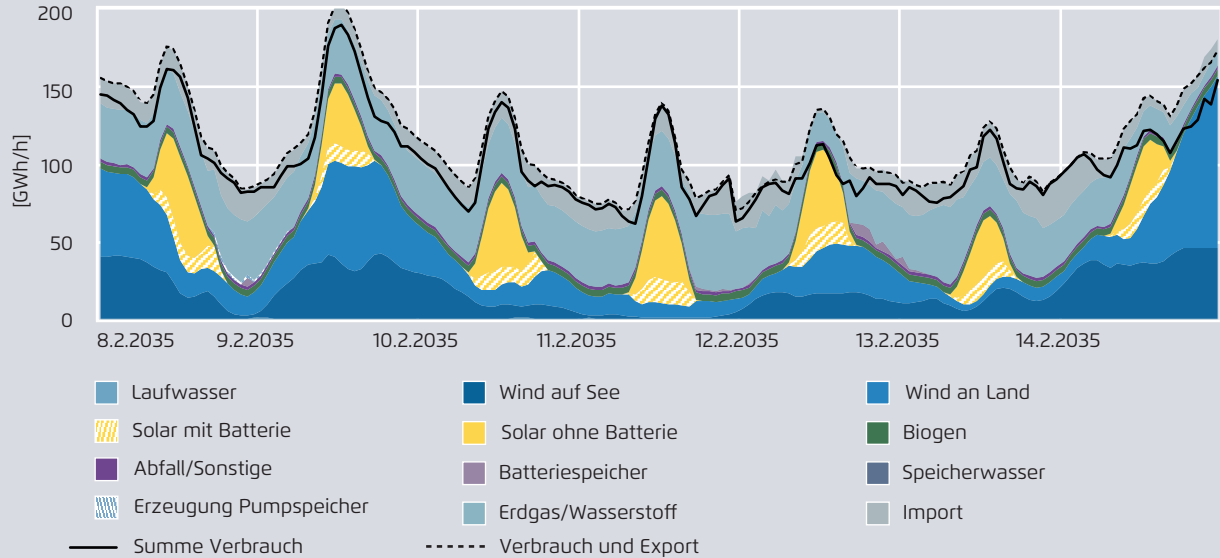
Stündliche Stromerzeugung und Stromnachfrage im Szenario KNS2035
