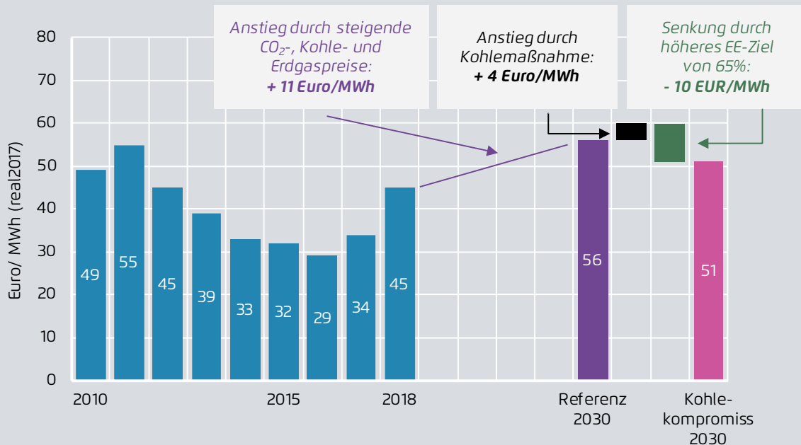
Abbildung 28: Entwicklung der Börsenstrompreise 2010 bis 2018 und 2030
