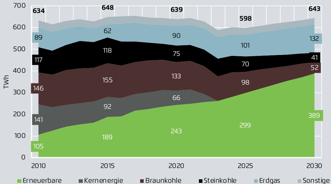
Abbildung 22: Bruttostromerzeugung 2010 - 2030 bei Umsetzung des Kohlekompromisses
