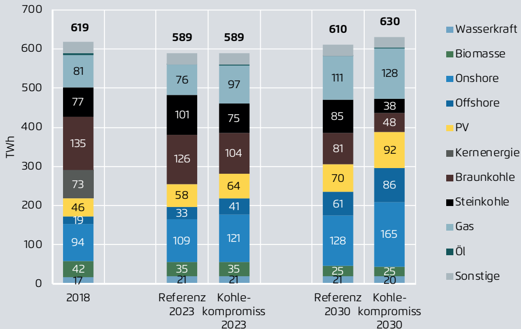
Abbildung 20: Stromerzeugung (netto) 2018, 2023 und 2030
