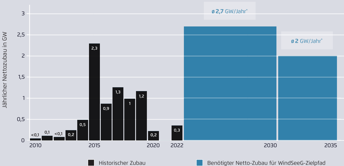
Historischer und zukünftig benötigter Wind-auf-See-Zubau für die WindSeeG-Ausbauziele
