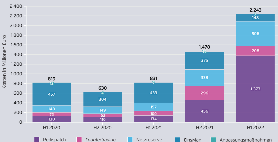
Kosten für Maßnahmen des Netzengpassmanagements 2020 bis 2022 (Halbjahre)
