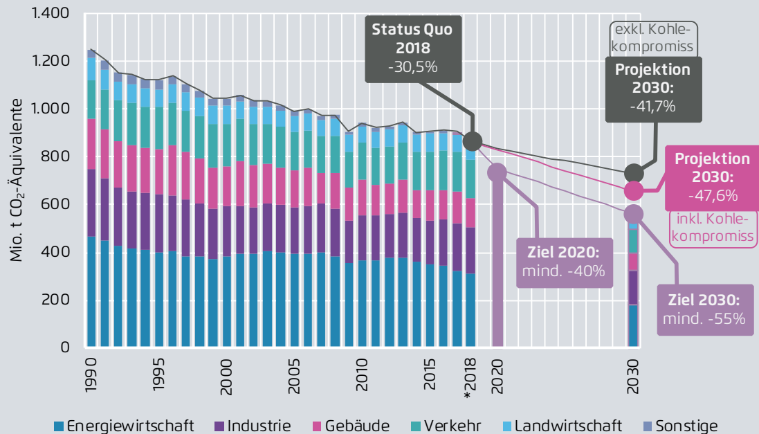
Abbildung Z-4: Treibhausgasemissionen nach Sektoren 1990 – 2018, Ziele und Projektion 2020 und 2030
