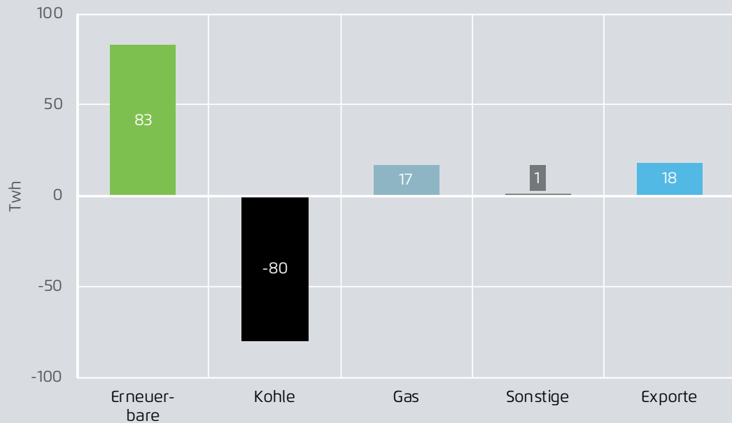
Abbildung 21: Differenz der Nettostromerzeugung zwischen Referenz- und Kohlekompromiss-Szenario 2030
