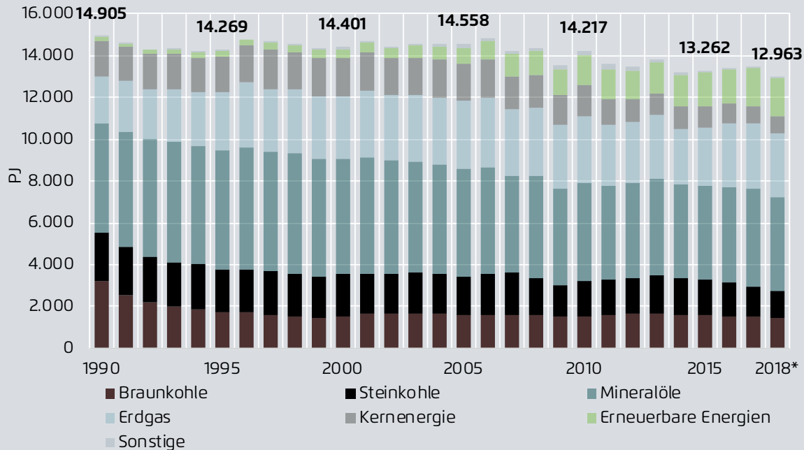
Abbildung 2: Primärenergieverbrauch 1990 - 2018
