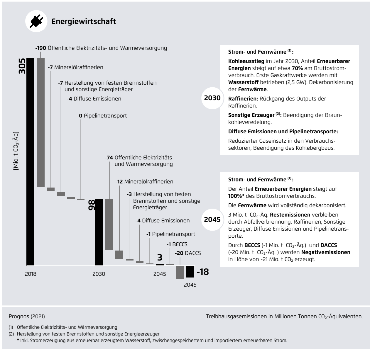
Reduktion der Treibhausgasemissionen in der Energiewirtschaft
