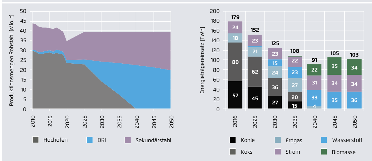
Rohstahlproduktion nach Routen und Energieträgereinsatz* in der Eisen- und Stahlindustrie Abbildung 26
