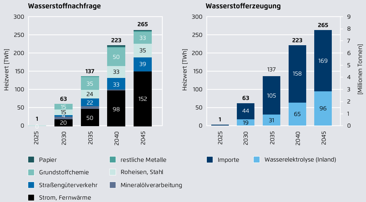
CO 2 -freie Wasserstoffherzeugung und -nutzung in Deutschland
