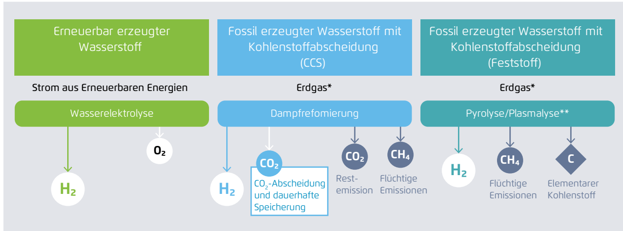
Treibhausgasfreie und -arme Verfahren zur Gewinnung von Wasserstoff
