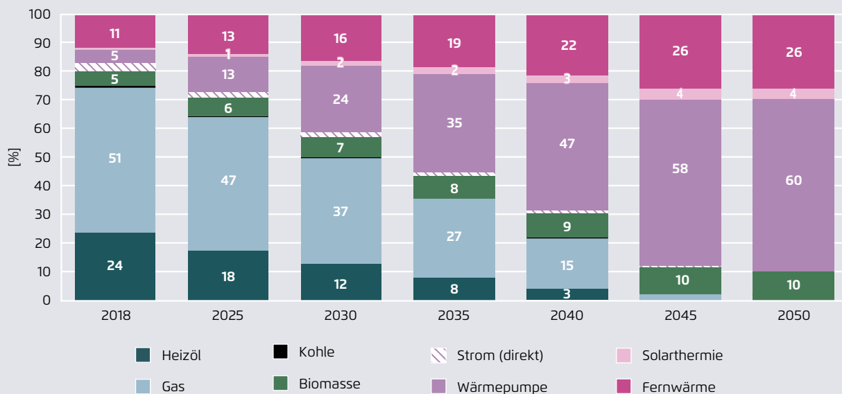
Beheizungsstruktur Wohnfläche
