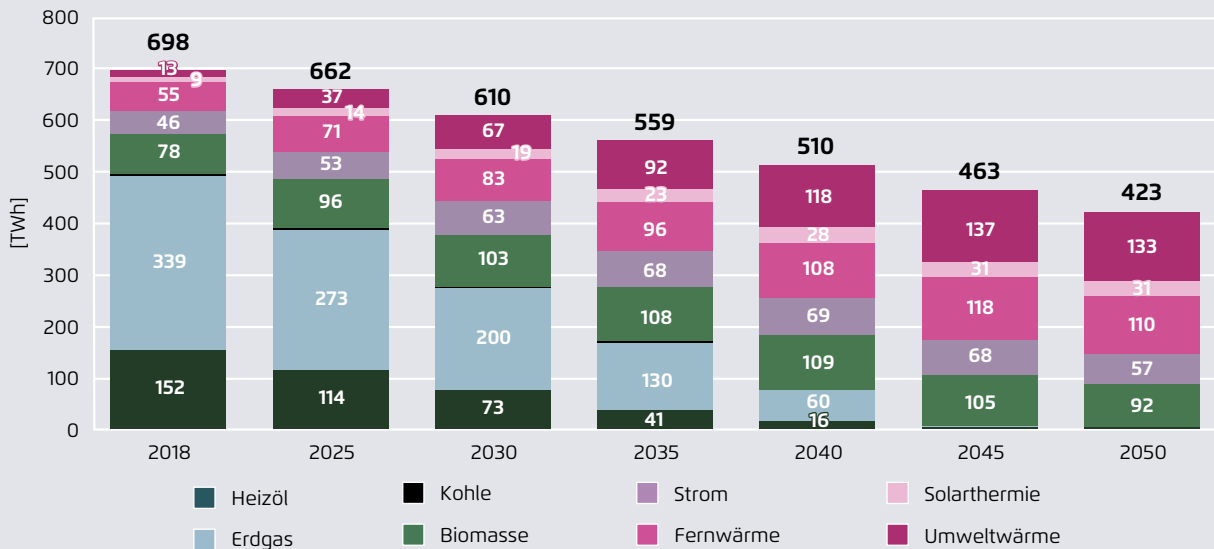
Gebäudesektor: Endenergieverbrauch für Wärme nach Energieträgern
