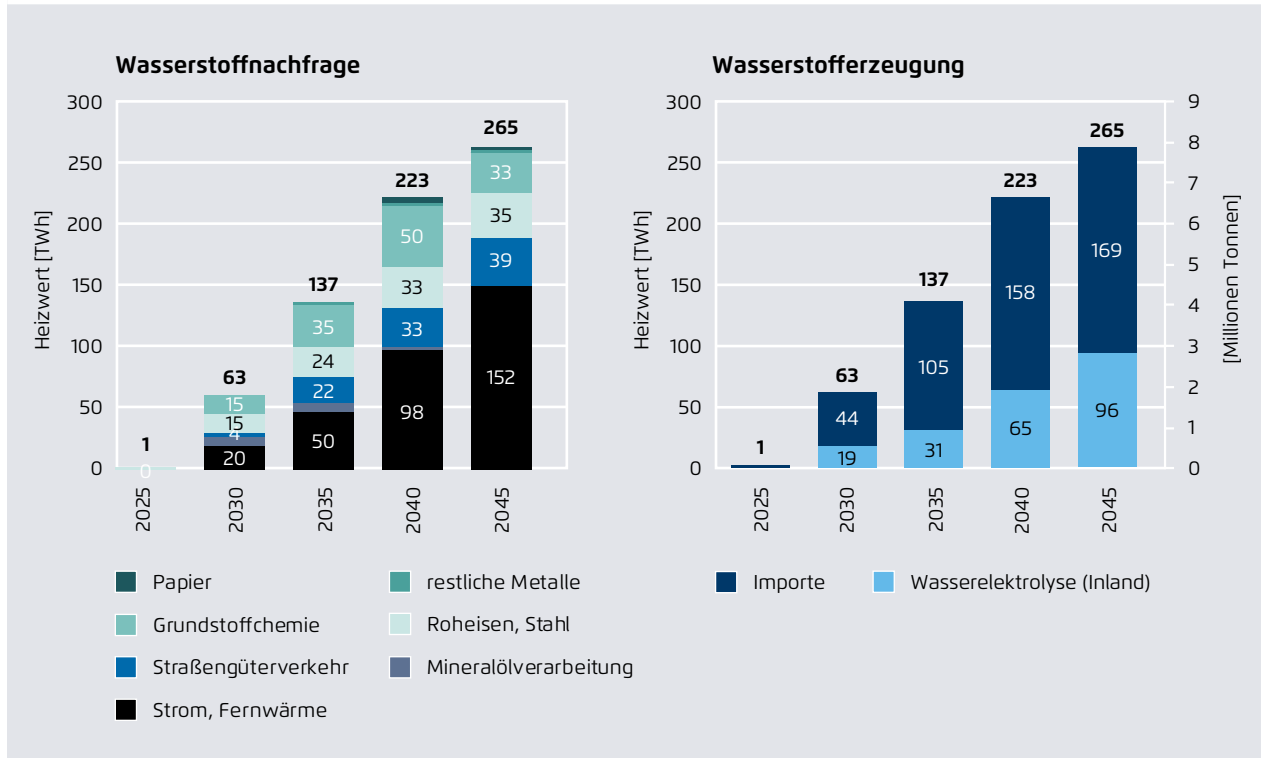
Treibhausgasfreie Wasserstoffnachfrage und Wasserstoffherzeugung
