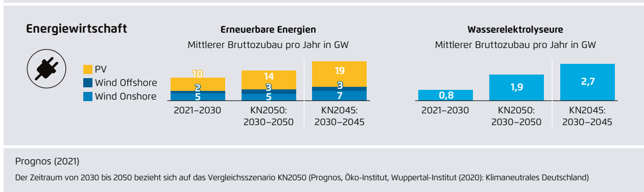
Umsetzungsgeschwindigkeit in den Szenarien KN2050 und KN2045
