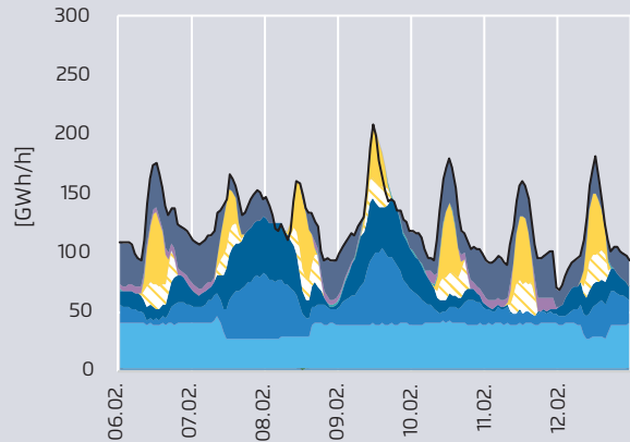
Erzeugung Winterwoche
