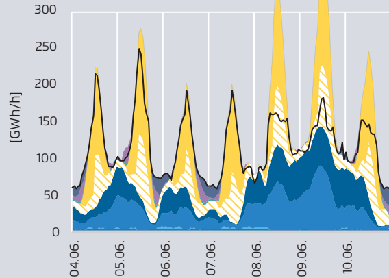
Erzeugung Sommerwoche
